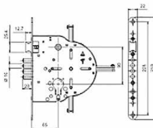
Zadbací zámek 265
