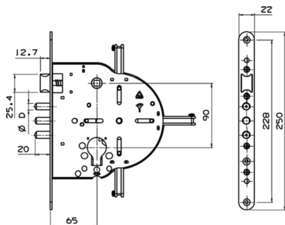
Zadbací zámek 235
