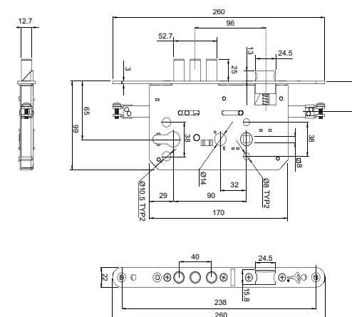
Zadbací zámek 212
